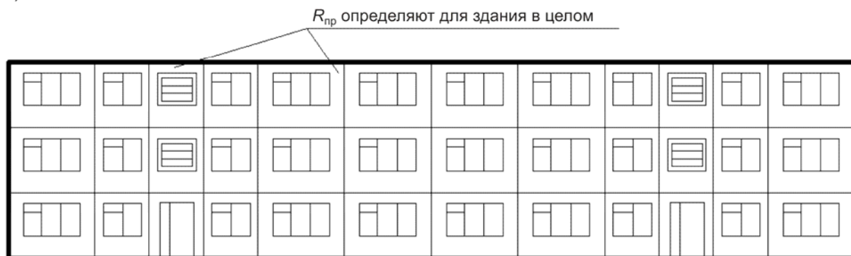
Рисунок 2 — Примеры определения приведенного сопротивления теплопередаче наружных стен многоэтажного жилого дома:
