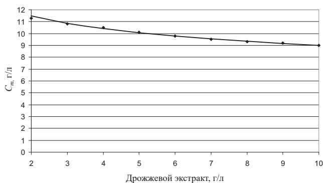
Рис. 5. Зависимость изменений величины ( C_m ) от концентрации дрожжевого экстракта (Ye) при фиксированных концентрациях глюкозы ( Gl=15\text{ г/л} ) и пептона ( Pe=4,5\text{ г/л} ) через 144 ч культивирования гриба Ph. impudicus
