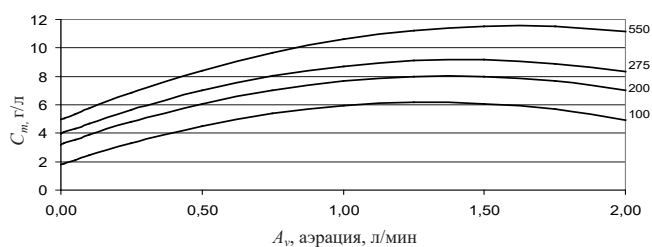
Рис. 3. Зависимости изменений величины ( C_m ) гриба Ph. impudicus от аэрации среды ( A_v ) и скорости вращения мешалки через 144 ч культивирования при температуре 28,0\text{ }^{\circ}\text{C} . 100, 200, 275, 550 — скорости вращения мешалки, об/мин
