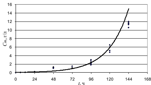
Рис. 6. Зависимость изменений величины ( C_m ) продуцента Ph. impudicus от времени культивирования ( t ) при фиксированных значениях факторов: T=28,0\text{ }^{\circ}\text{C} ; pH=5,0 ; A_v=1,75\text{ л/мин} ; V=550\text{ об/мин} ; Pe=4,5\text{ г/л} ; Gl=15\text{ г/л} ; Ye=2,5\text{ г/л}
